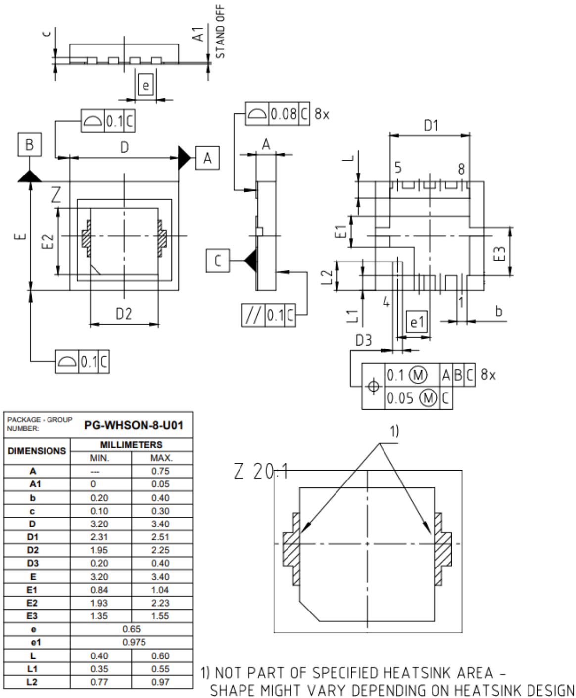
图 1 PG-WHSON-8 外形图，尺寸单位为毫米
