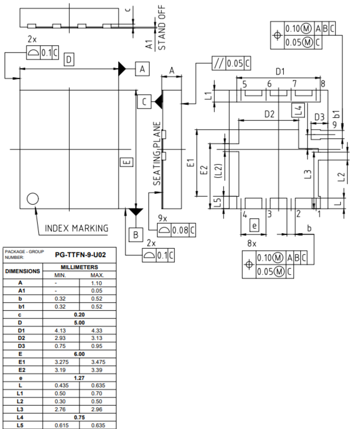
图 1 PG-TTFN-9 外形图，尺寸单位为毫米
