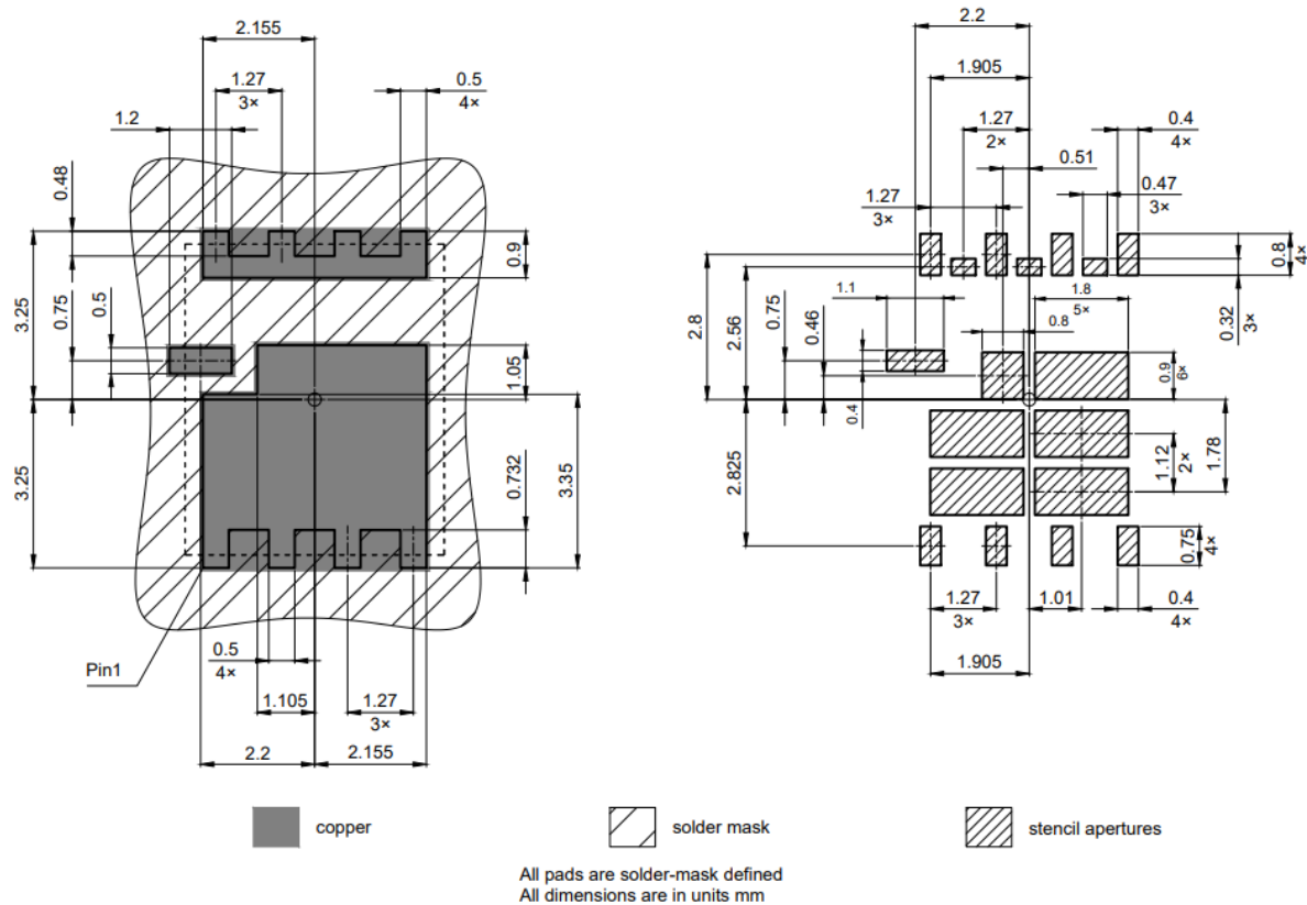
图 2 PG-WHTFN-9封装图, 尺寸单位为毫米
