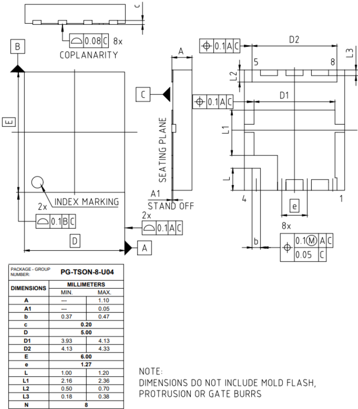
图 1 PG-TSON-8 外形图, 尺寸单位为毫米
