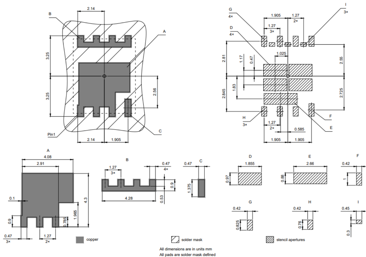
图 2 PG-WHSON-8 封装图, 尺寸单位为毫米
