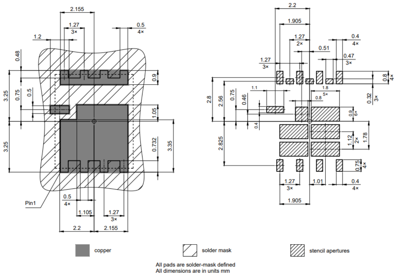
图 2 PG- WHTFN- 9封装图，尺寸单位为毫米
