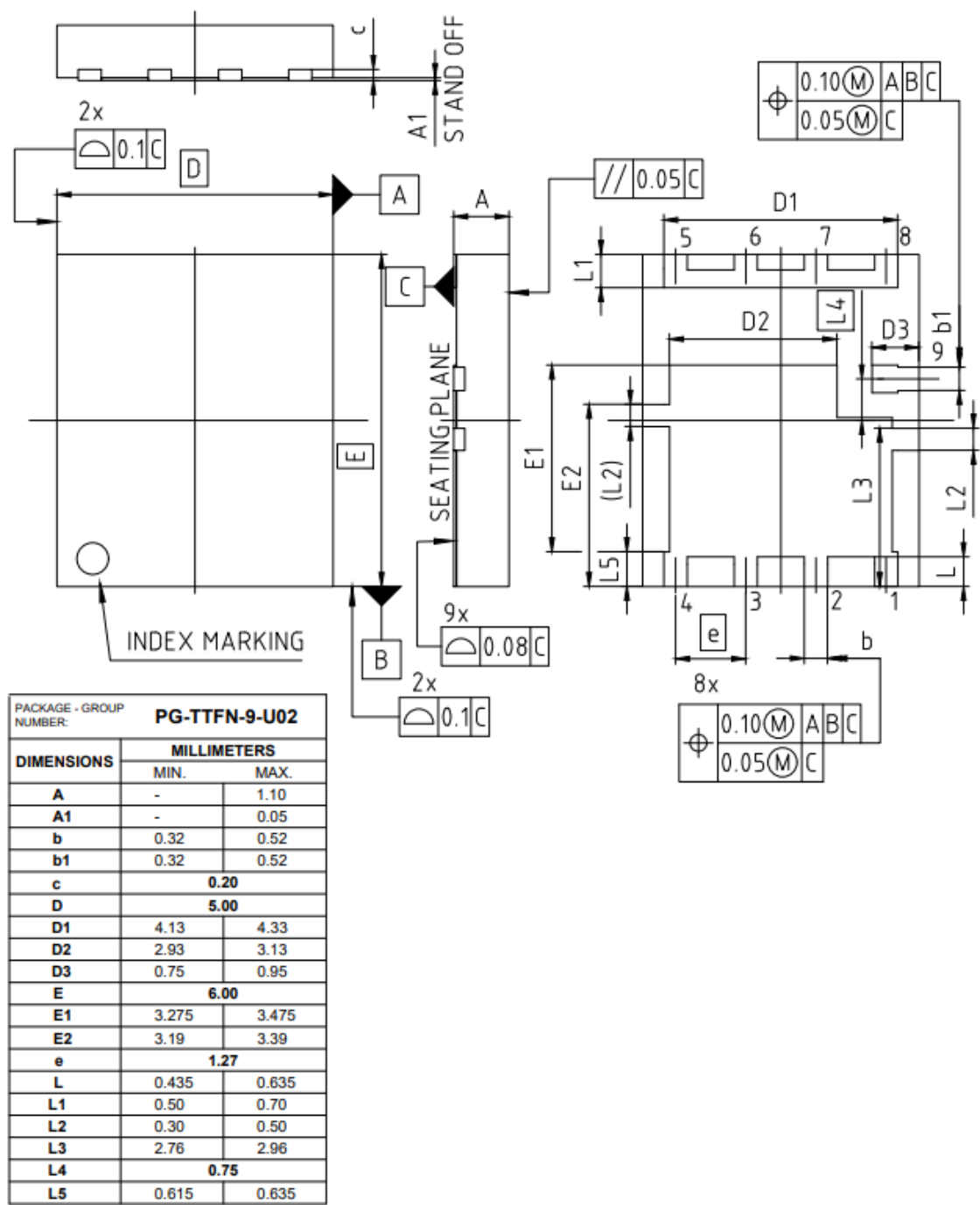
图 1 PG-TTFN-9 外形图，尺寸单位为毫米
