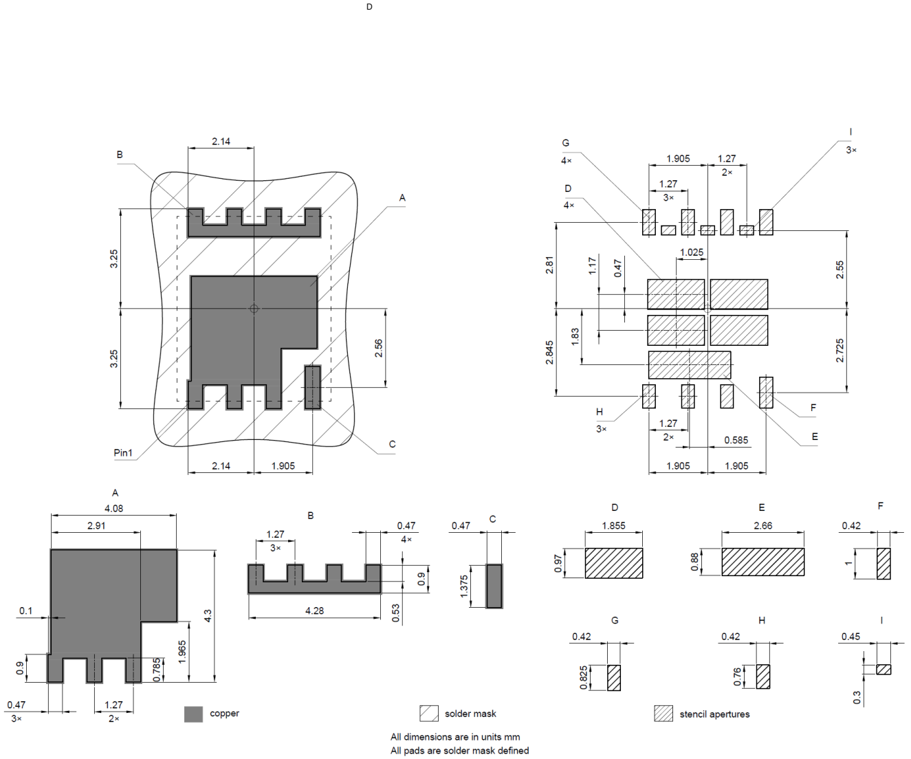
图 2 PG-WHSON-8 封装图，尺寸单位为毫米
