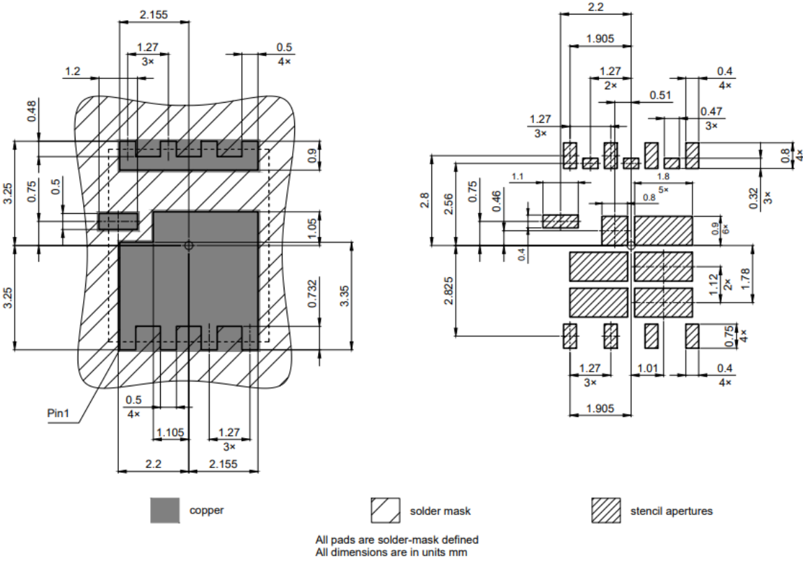
图 2 PG- WHTFN- 9封装图，尺寸单位为毫米
