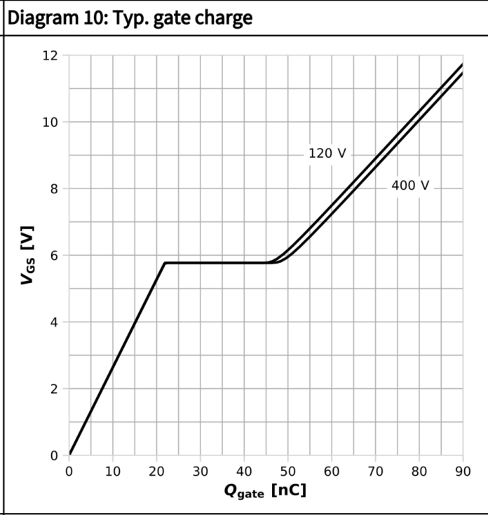
V_{GS} = f(Q_{gate}) ; I_D = 13.5 A pulsed; parameter: V_{DD}
