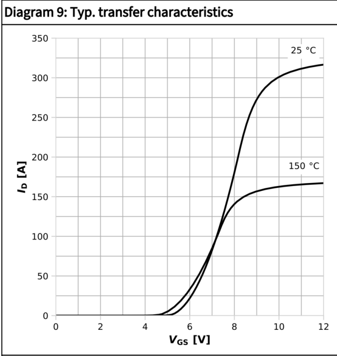
I_D = f(V_{GS}) ; V_{DS} = 20V ; parameter: T_j
