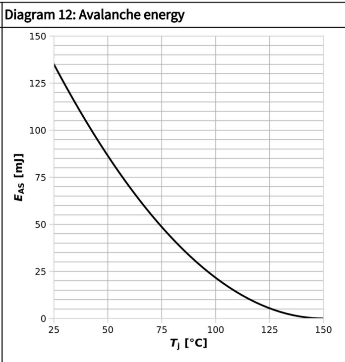
E_{AS} = f(T_j) ; I_D = 4.9 A ; V_{DD} = 50 V
