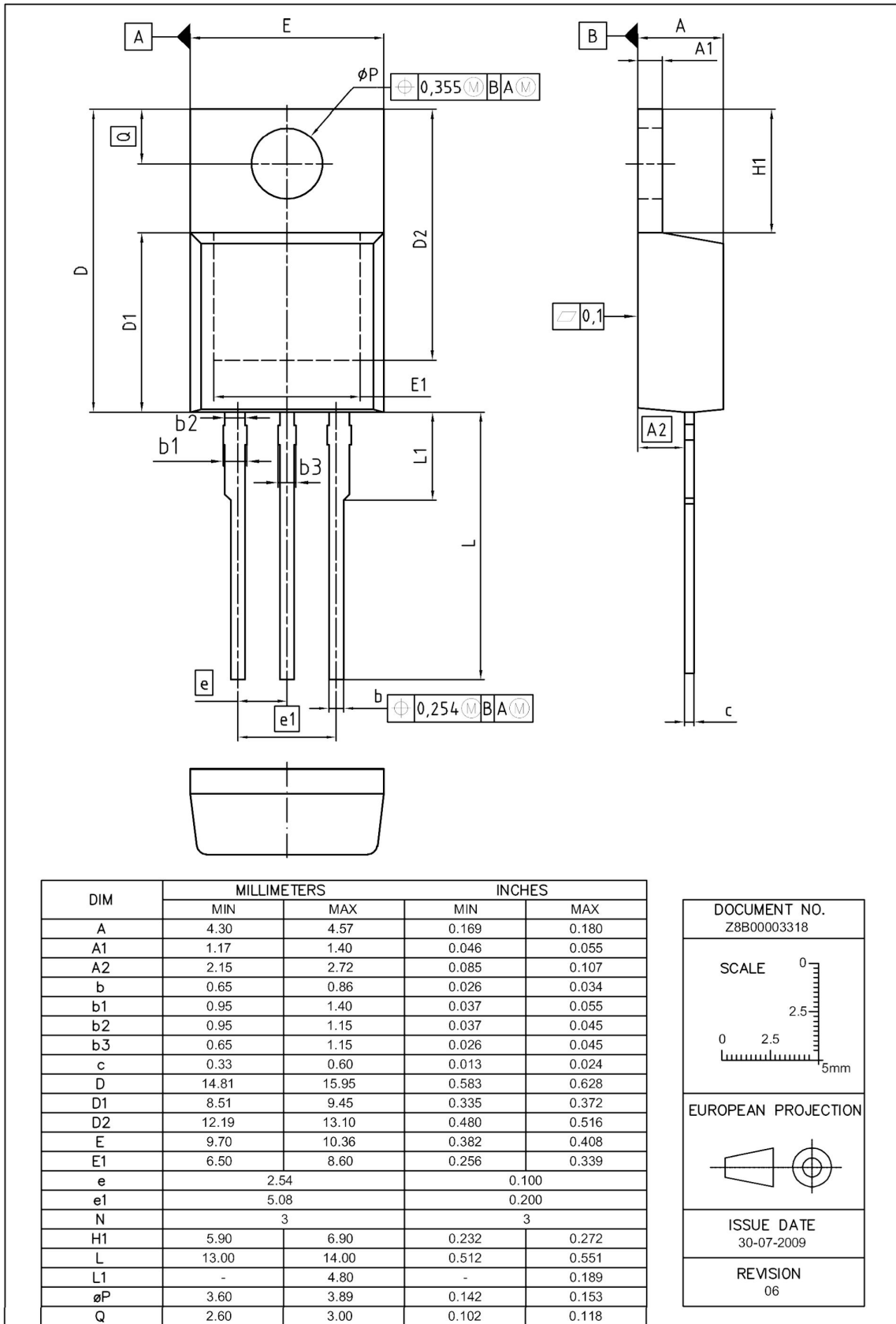
图 3 PG-TO 220 封装外形，尺寸单位为毫米/英寸
