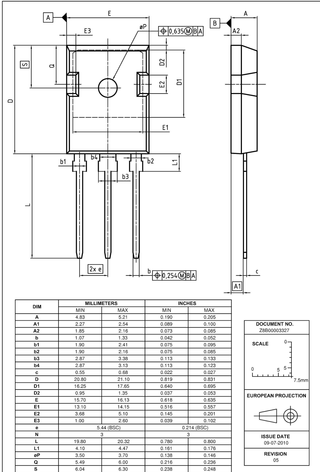
图1 PG-TO 247 封装外形，尺寸单位：毫米/英寸
