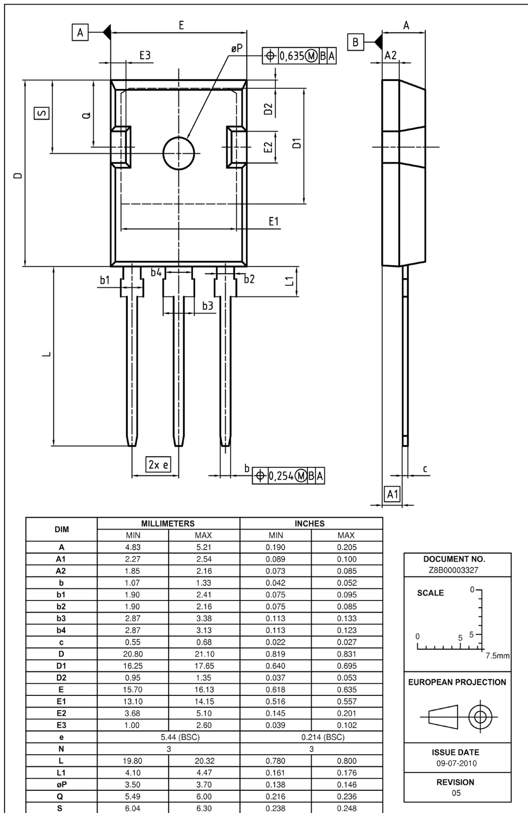
图 1 PG-TO 247 封装外形，尺寸单位：毫米/英寸
