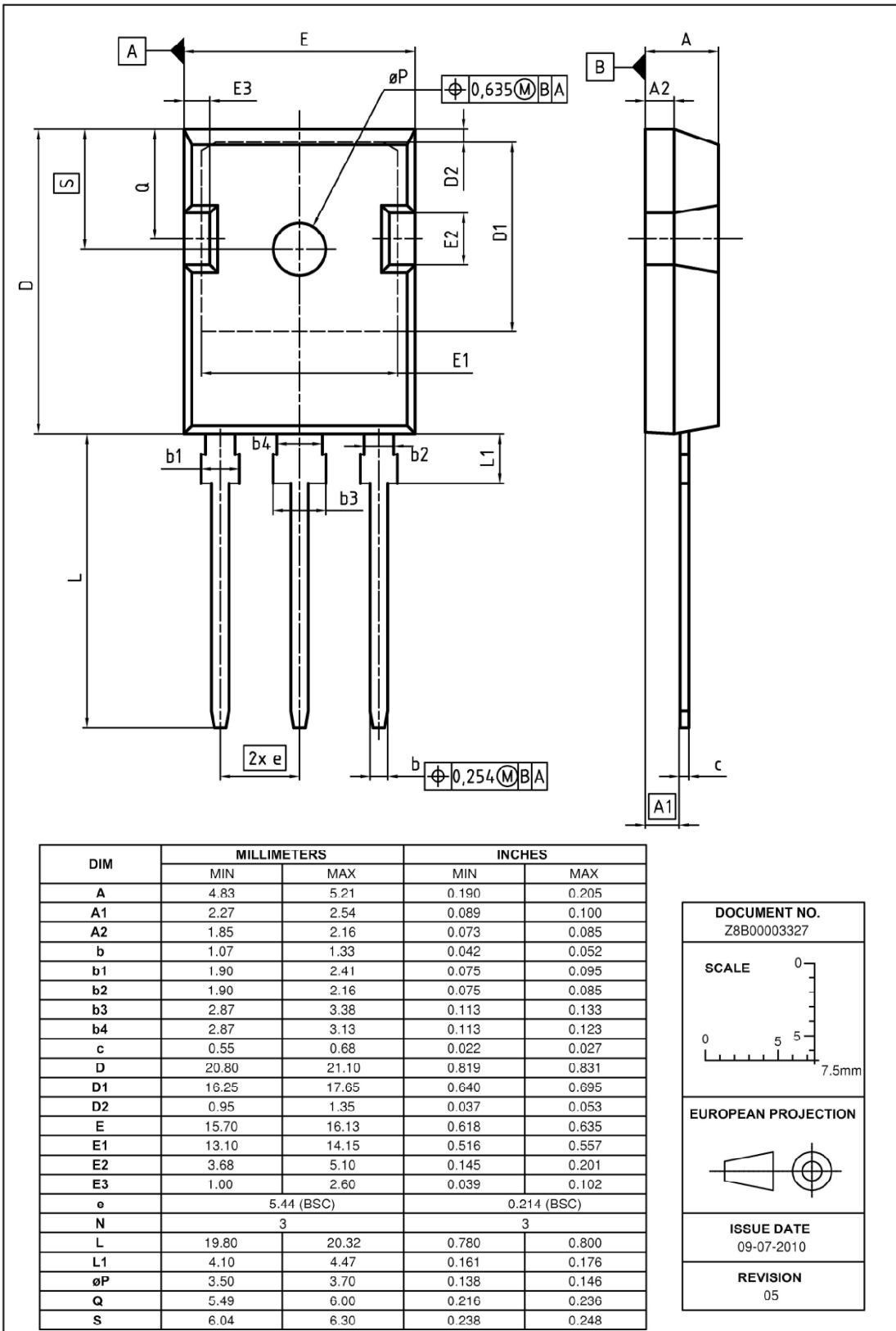
图 1 PG-TO 247-3 外形, 尺寸单位: 毫米/英寸
