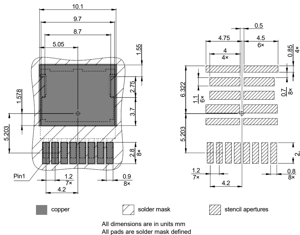
图 2 PG- HSOG 8 外形图, 尺寸单位为毫米
