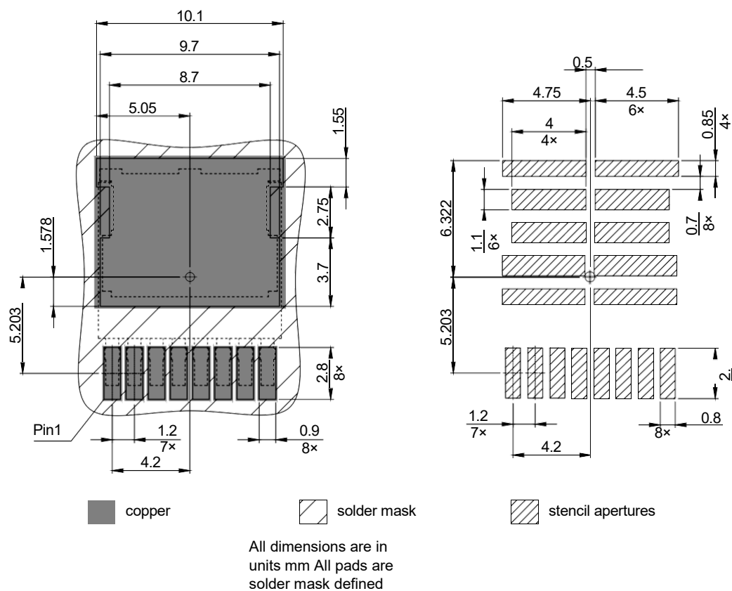
图 2 PG-HSOG-8 外形图, 尺寸单位为毫米
