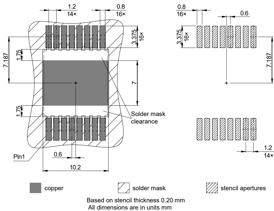
图 2 PG-HDSOP-16 外形图, 尺寸单位为毫米
