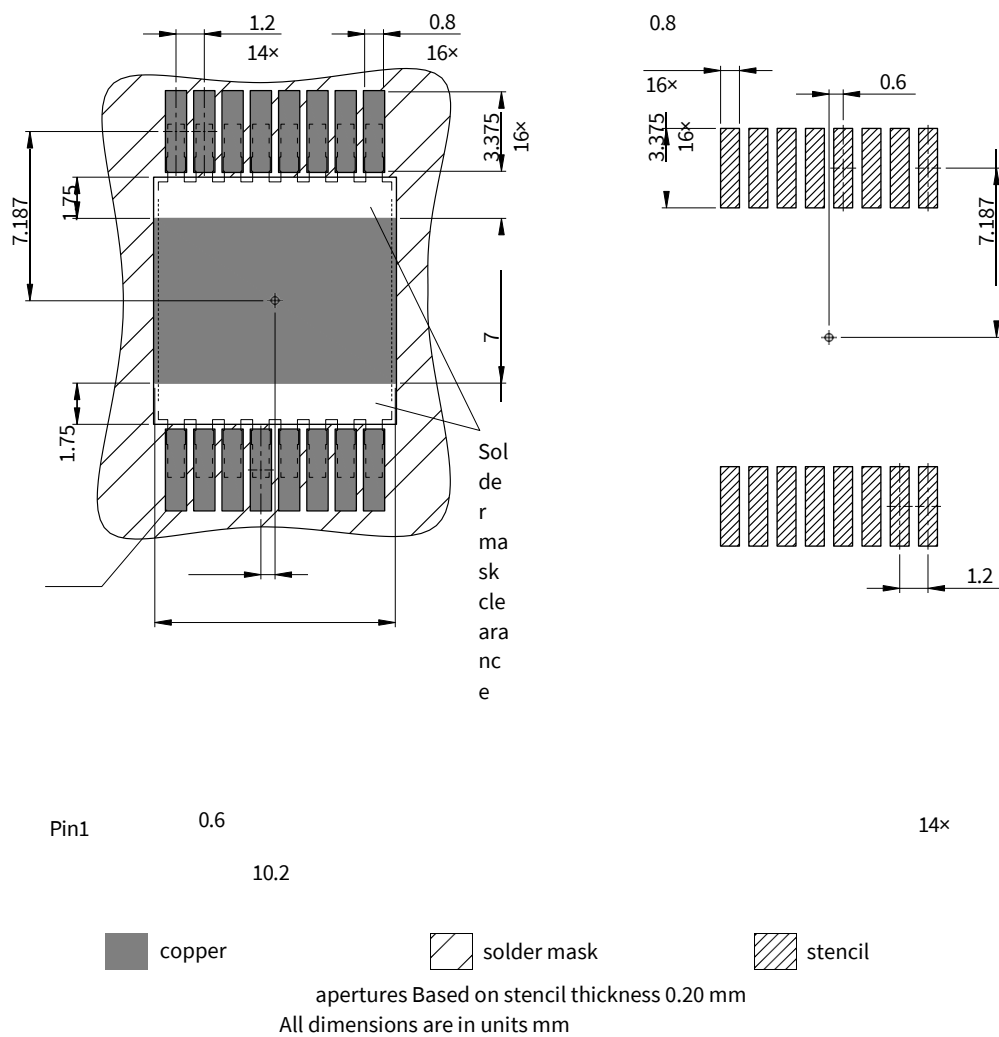
图 2 封装外形尺寸 (PG-HDSOP-16)，尺寸单位为毫米
