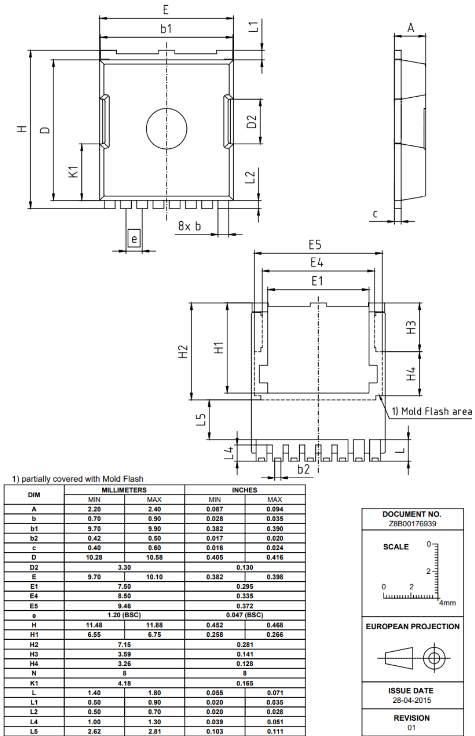
图 1 PG-HSOF-8 外形图，尺寸单位为毫米/英寸
