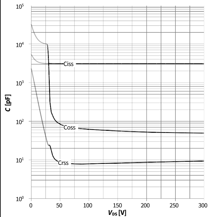
Diagram 15: Typ. 电容值
