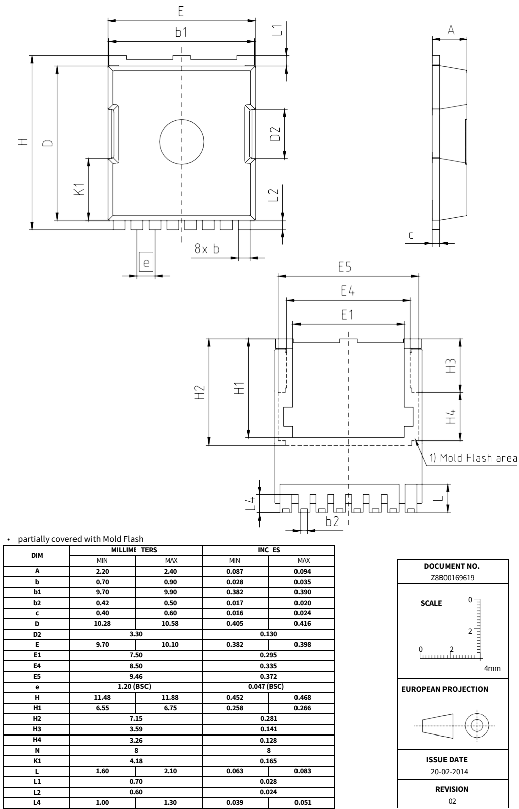
图 1 PG-HSOF-8 外形图，尺寸单位为毫米/英寸
