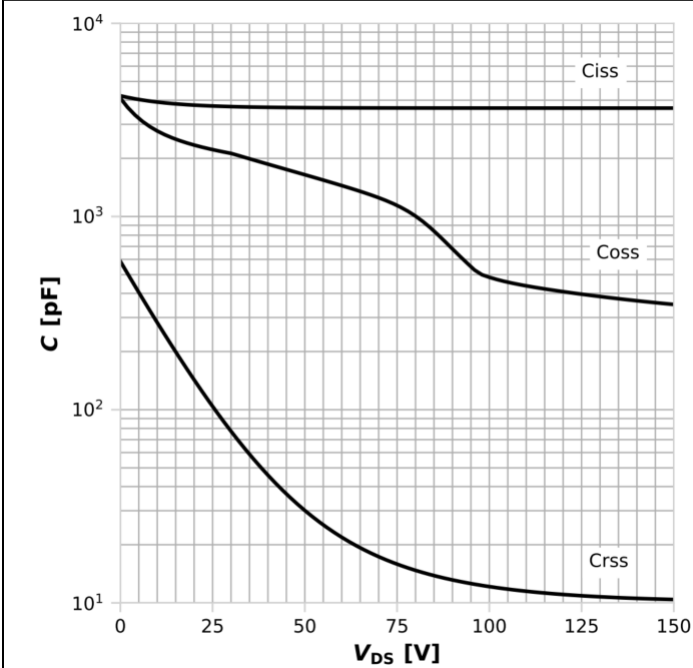
图 11: 典型电容值
