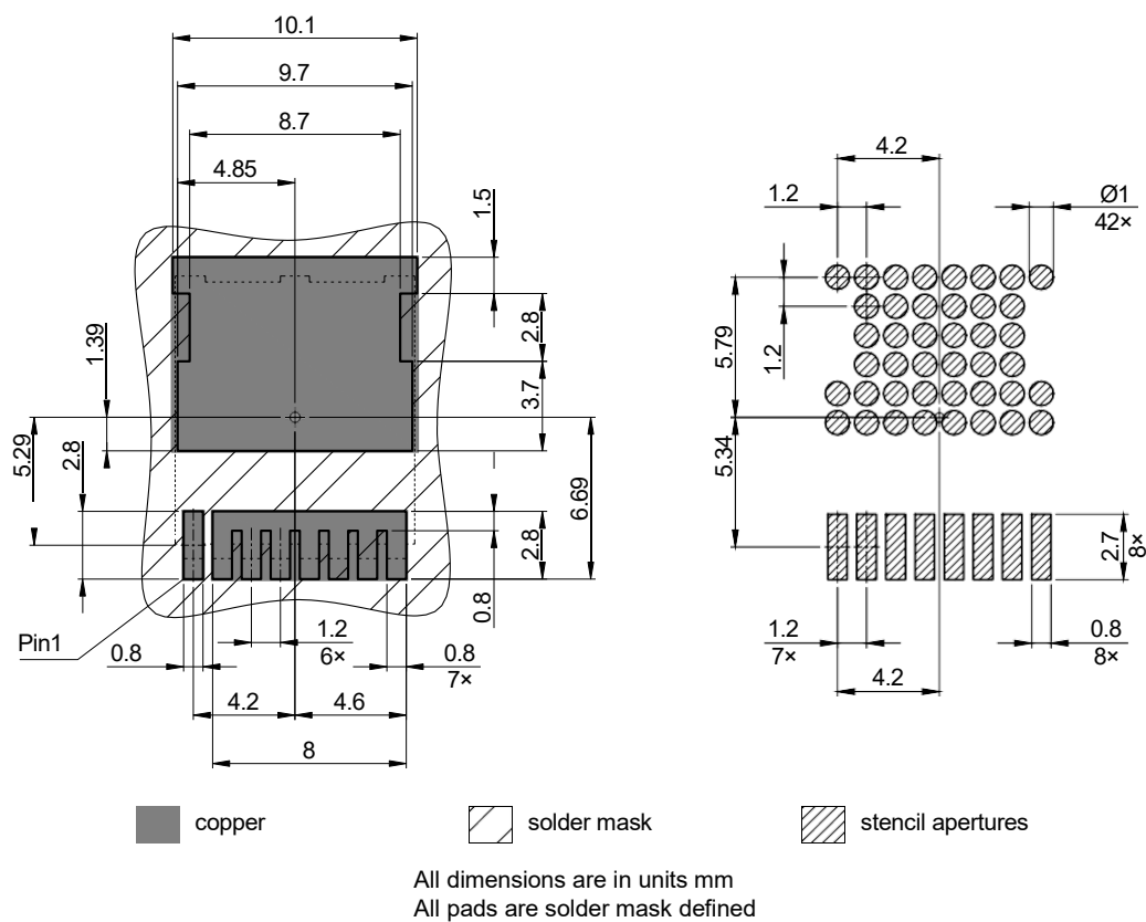
图 2 PG-HSOF-8 外形图, 尺寸单位为毫米
