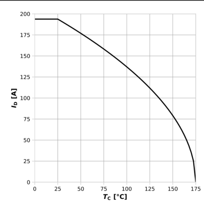
图2：漏极电流
