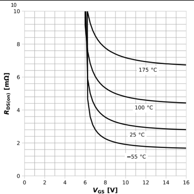
图 8: 典型漏源导通电阻
