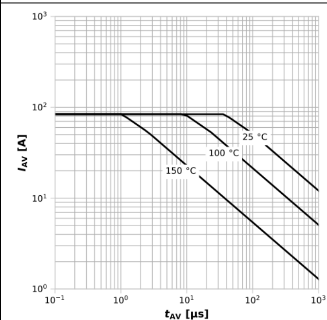
图 13: 雪崩特性
