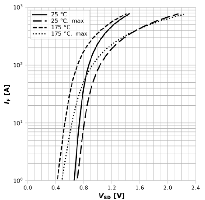
图 12: 反向二极管的正向特性
