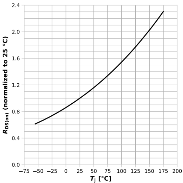
图 9: 归一化漏通电阻
