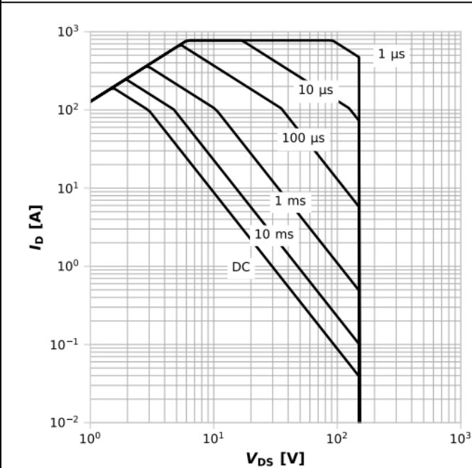
图3：安全操作区
