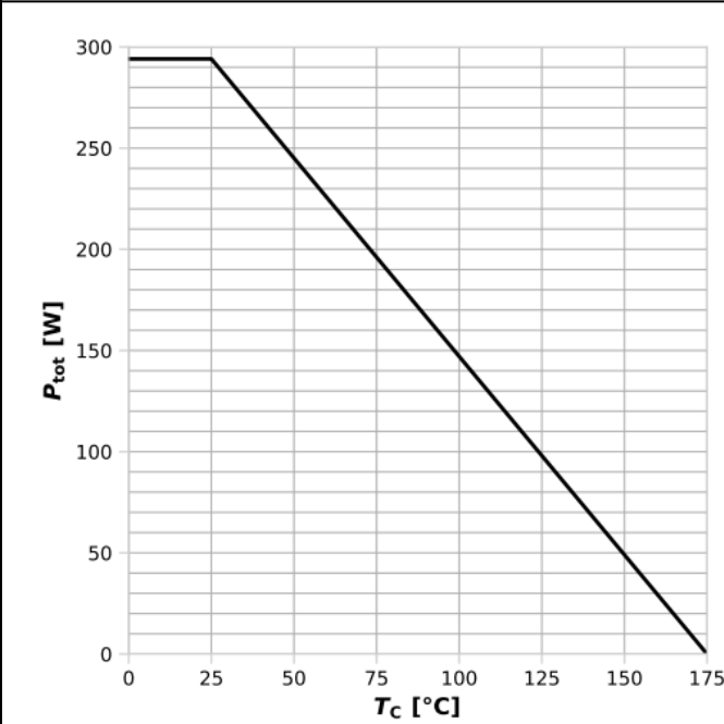
图1：功率耗散
