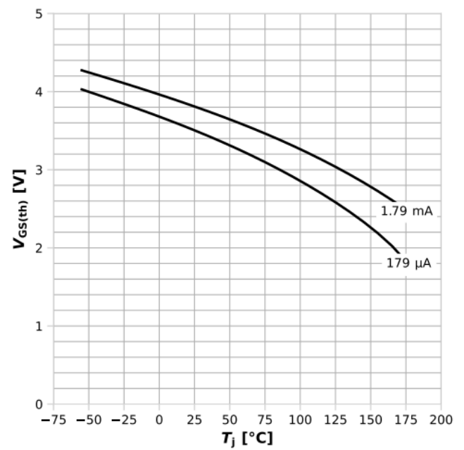
图 10: 典型栅极阈值电压
