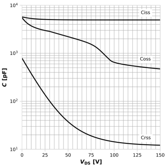
图 11: 典型电容值
