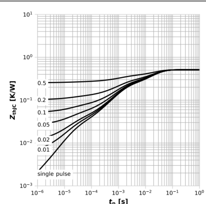
图4：最大瞬态热阻抗
