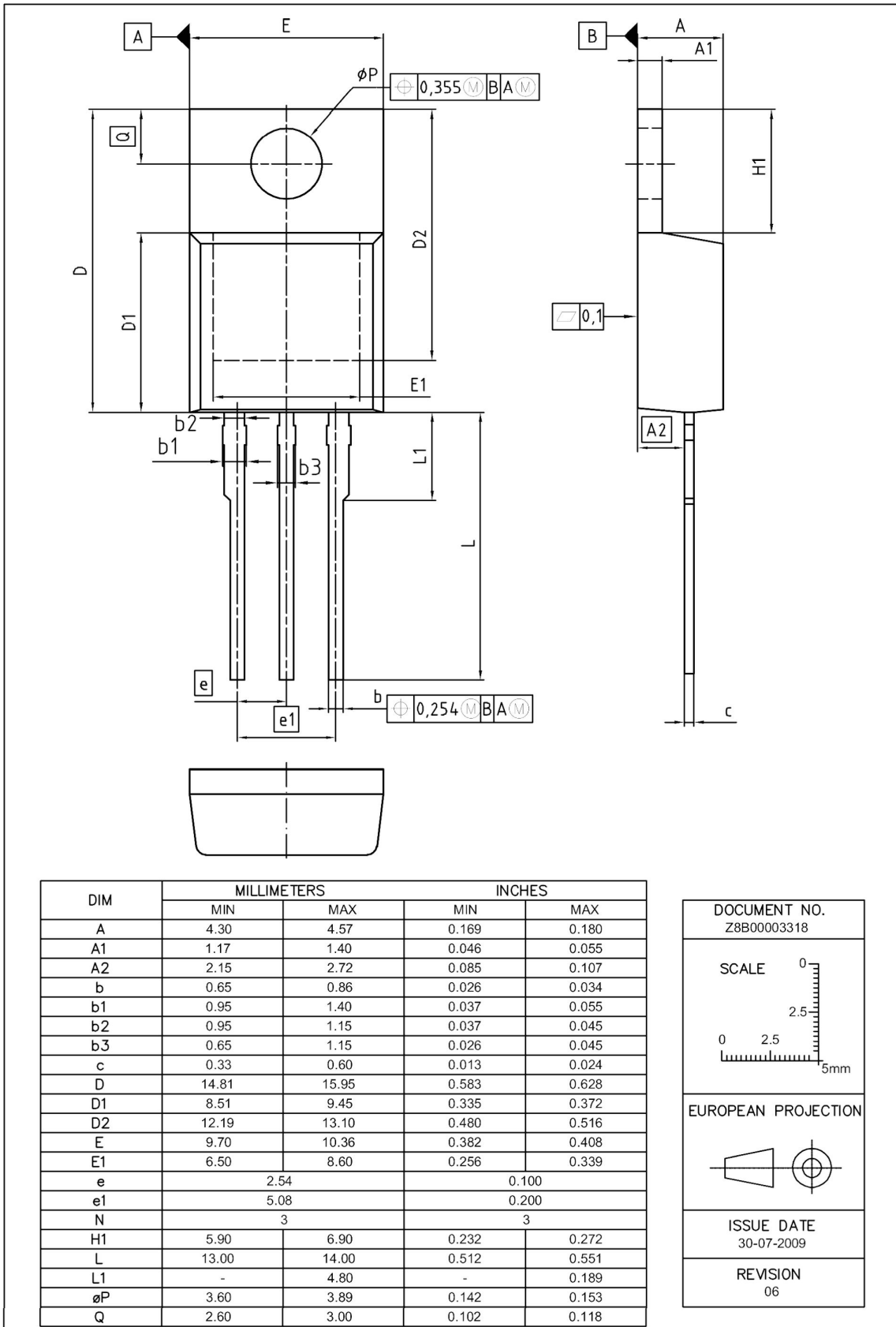
图 1 PG-TO 220-3 外形图，尺寸单位为毫米/英寸
