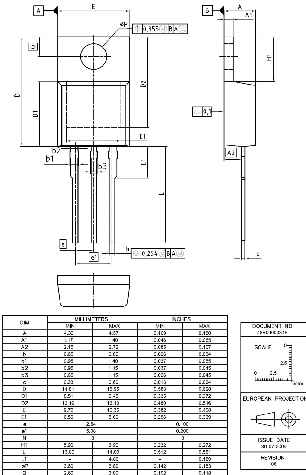
图 1 PG-T0220-3 外形图，尺寸单位为毫米/英寸
