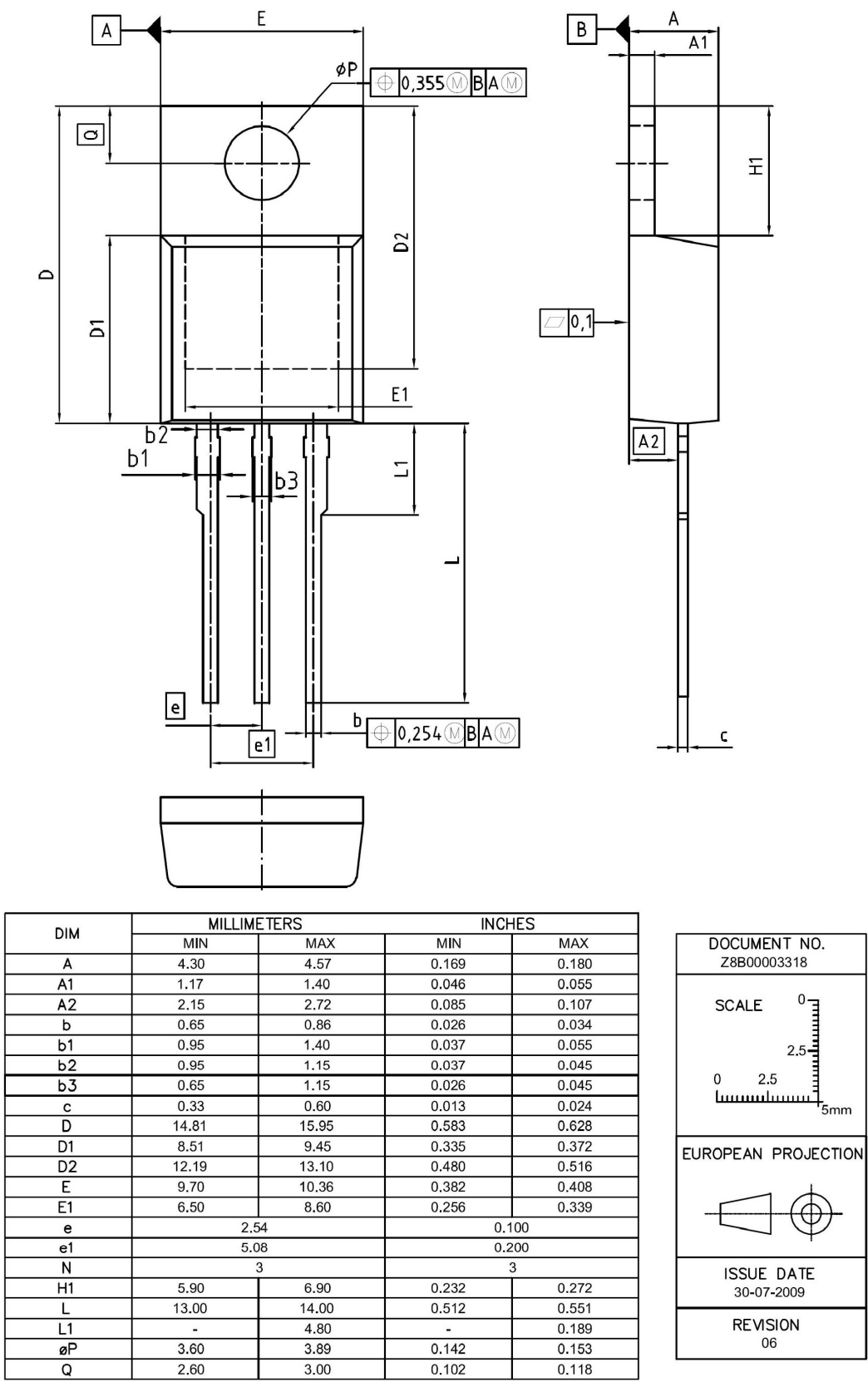
图 1 PG-T0220-3 外形图, 尺寸单位为毫米/英寸
