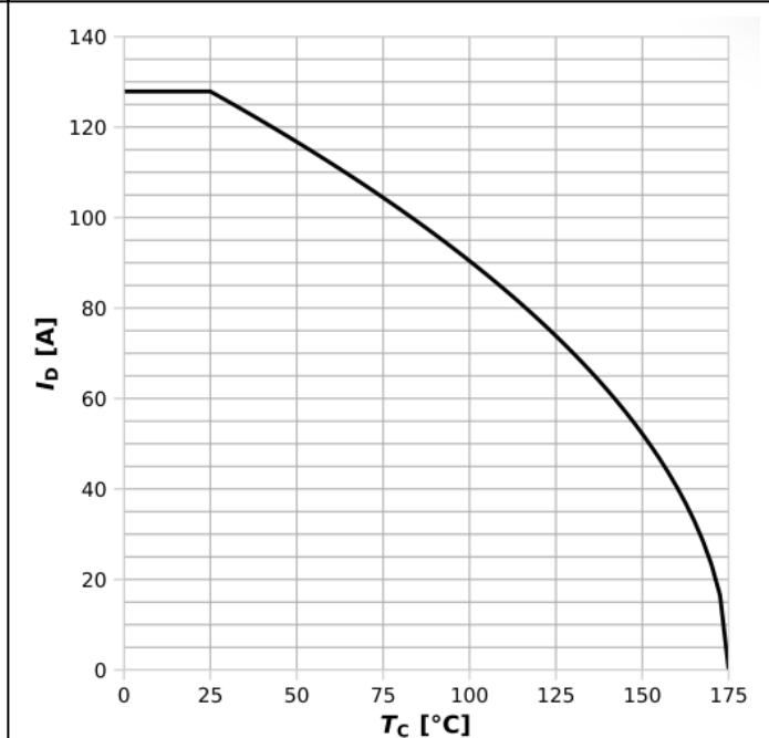
图 2: 漏极电流
