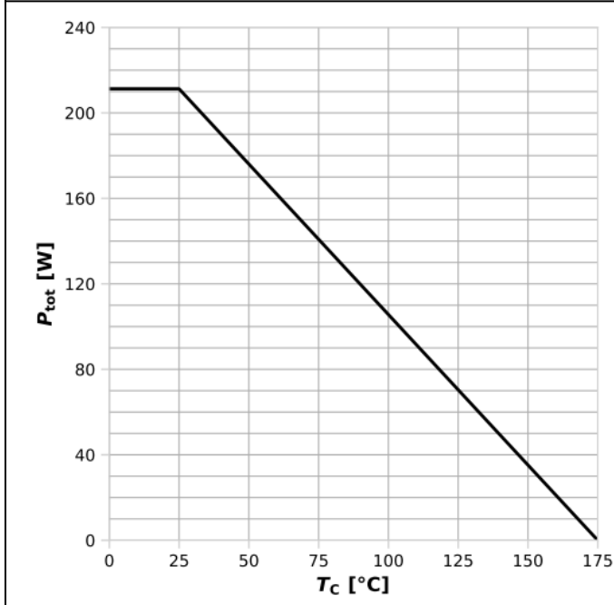
图 1: 功率耗散
