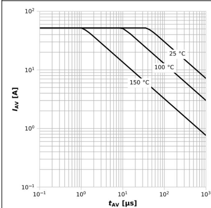
图 13: 雪崩特性
