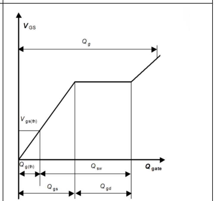
栅极充电波形
