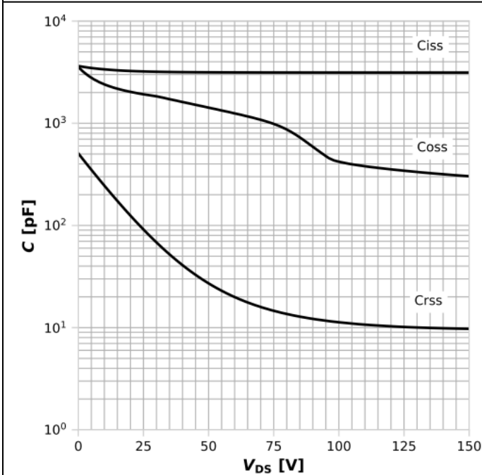
图 11: 典型电容值
