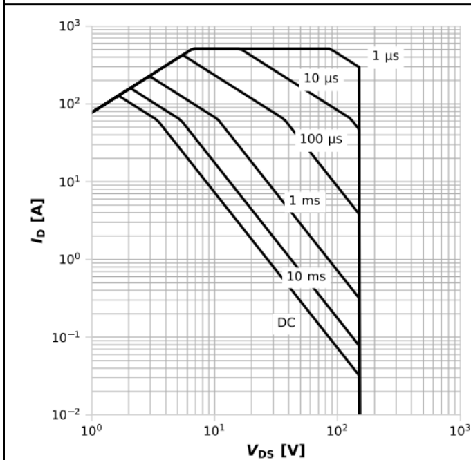
图 3: 安全操作区
