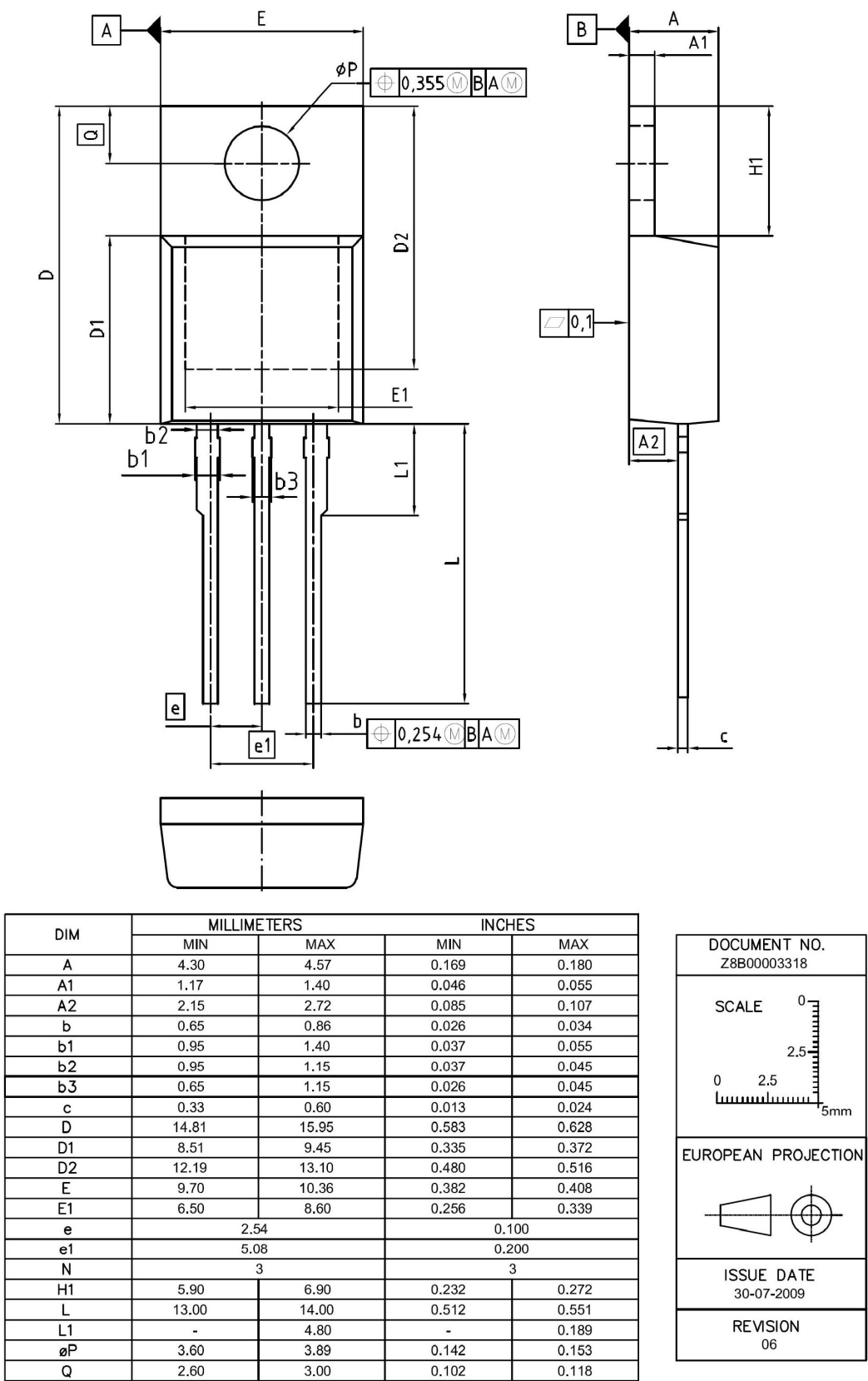
图 1 PG-TO 220-3 外形图，尺寸单位为毫米/英寸
