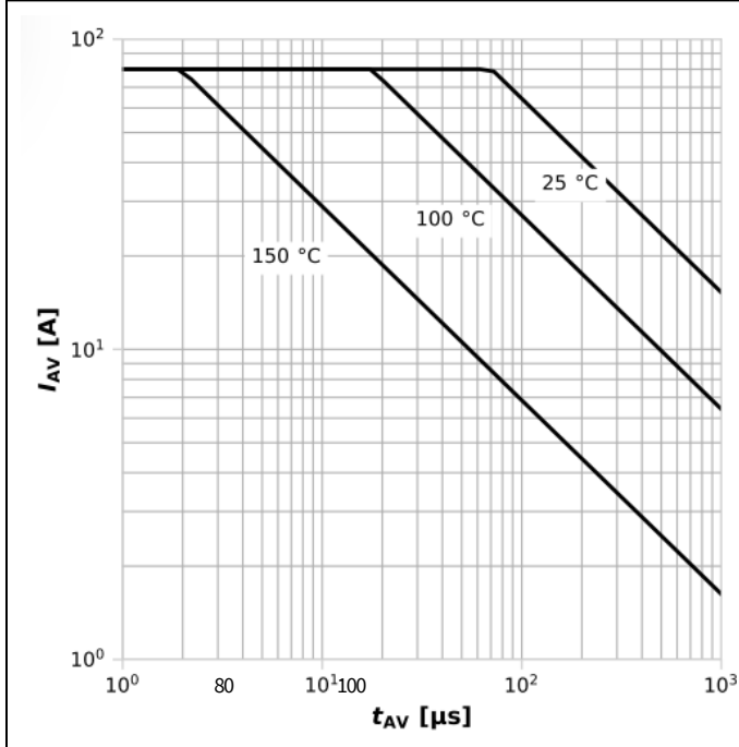
图 13: 雪崩特性
