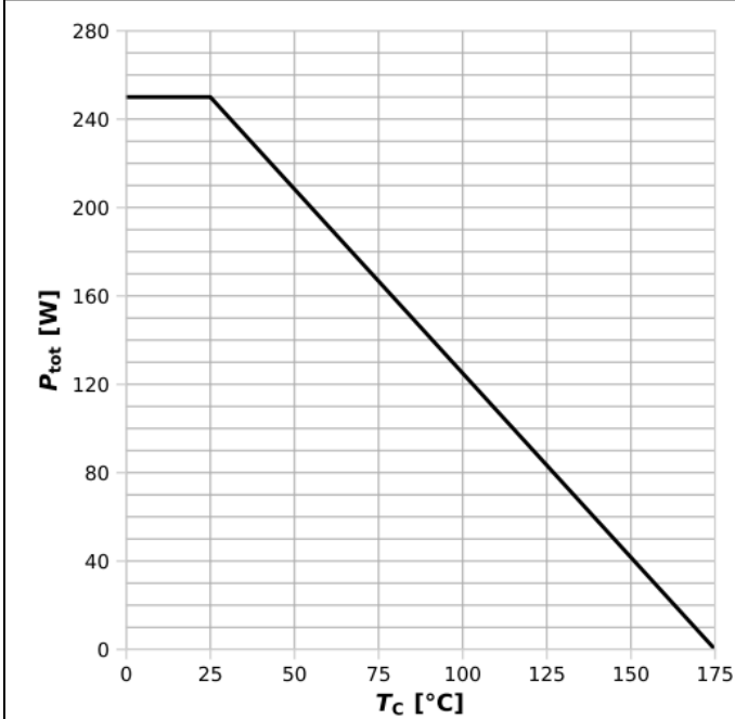
图 1: 功率耗散
