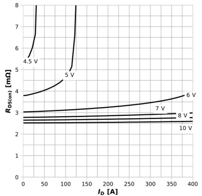
图 6: 典型漏源导通电阻
