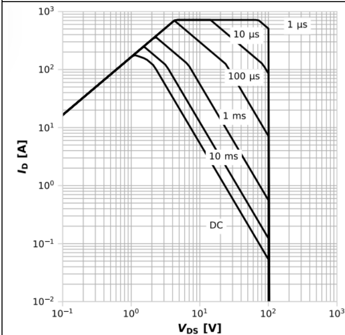
图 3: 安全操作区
