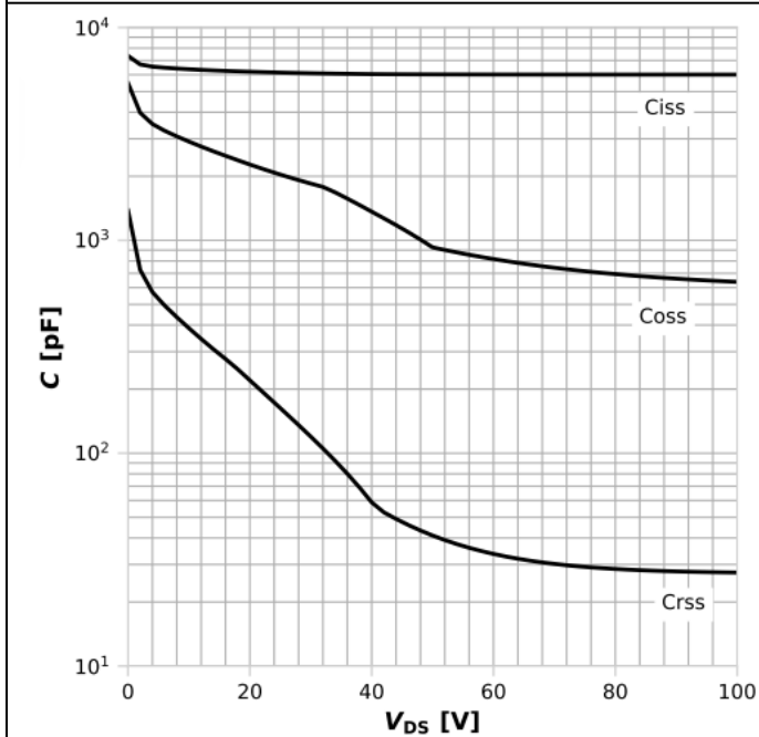
图 11: 典型电容值
