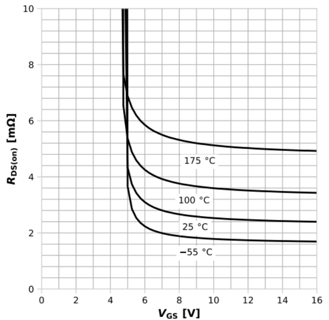
图 8: 典型漏源导通电阻
