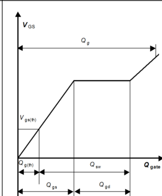
栅极充电波形
