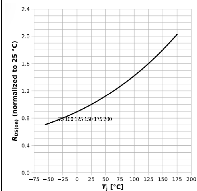
图 9: 归一化漏通电阻
