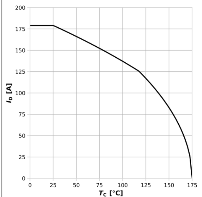
图 2: 漏极电流
