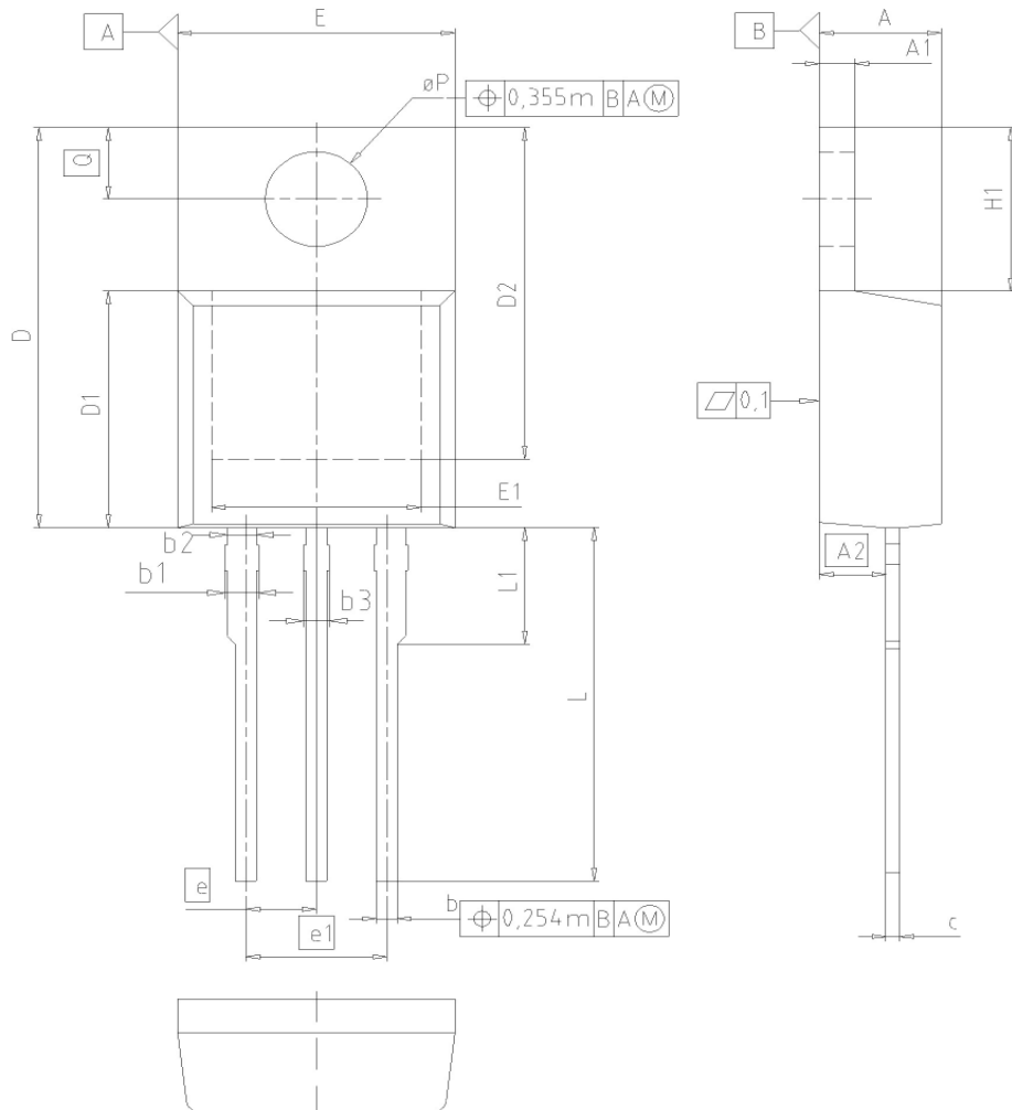
PG-TO220-3: 外形图
