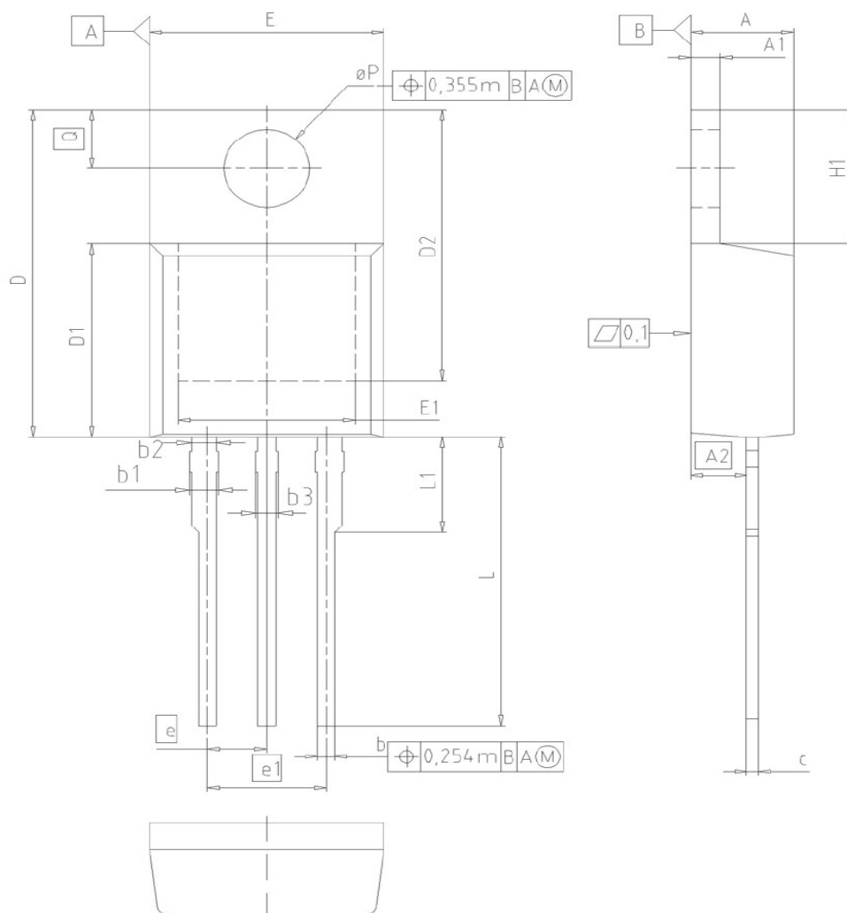
PG-TO220-3: 外形图
