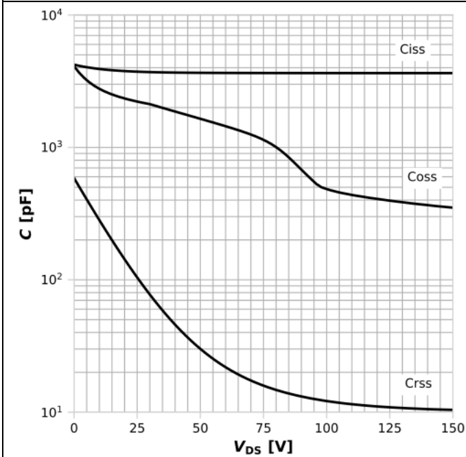
图11：典型电容值
