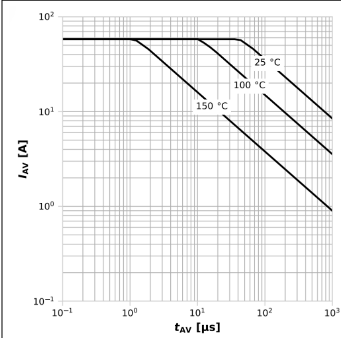
图 13: 雪崩特性
