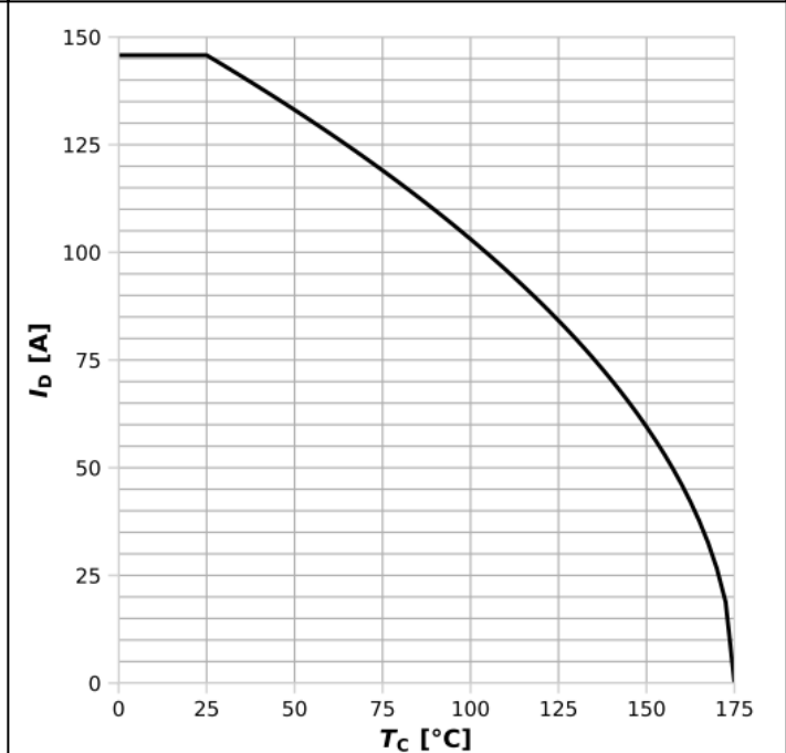
图2: 漏极电流
