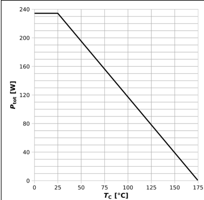
图1: 功率耗散
