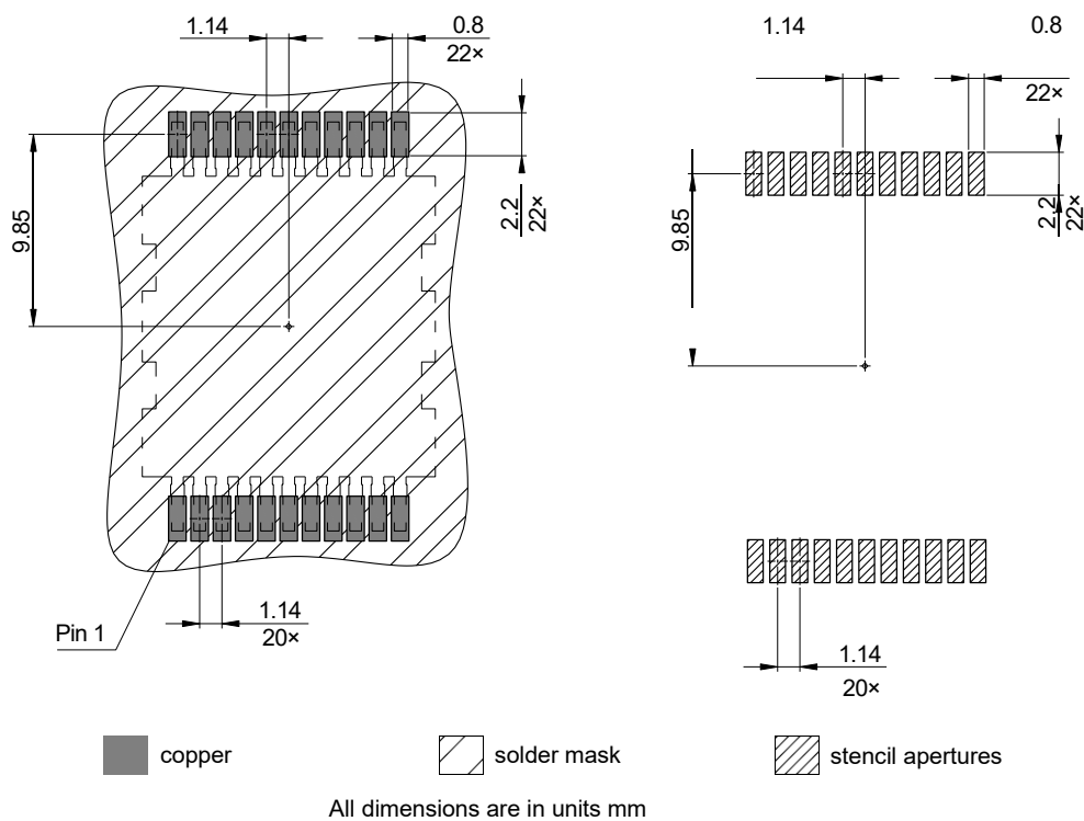
图 2 PG-HDSOP-22 封装图，尺寸单位为毫米
