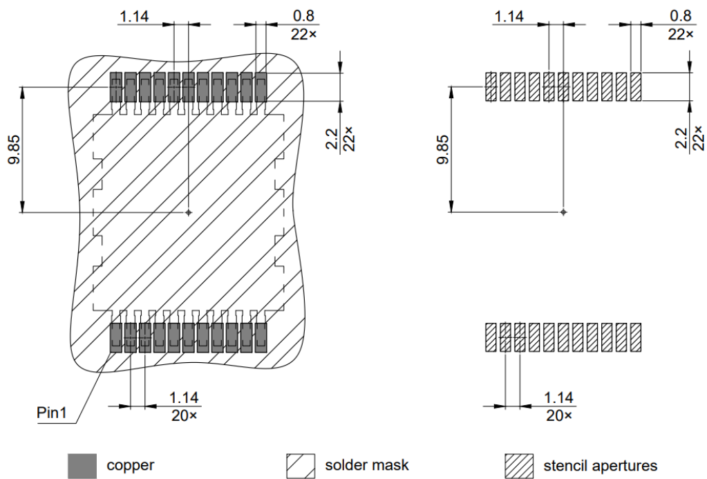
图 2 PG-HDSOP-22 外形图，尺寸单位为毫米
