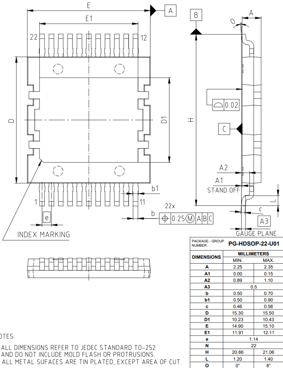
图 1 PG-HDSOP-22 外形图，尺寸单位为毫米
