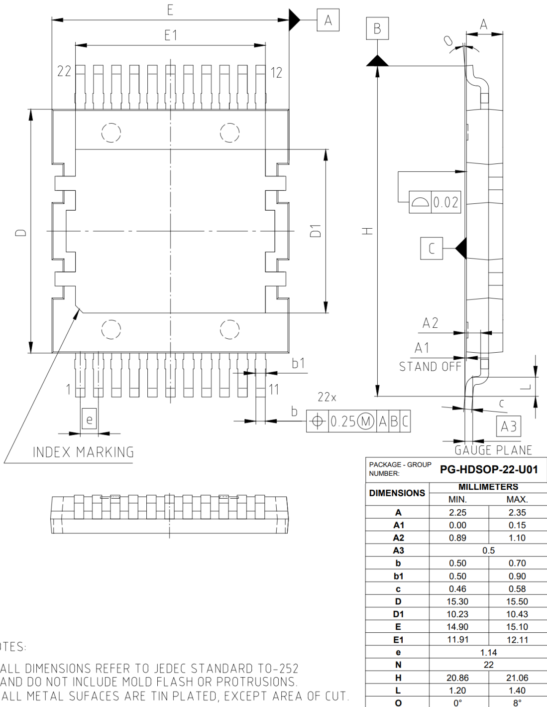
图 1 PG-HDSOP-22 外形图，尺寸单位为毫米
