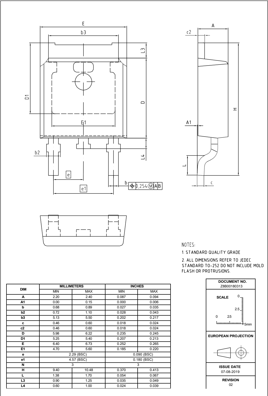
图 1 PG-TO 252-3 外形图，尺寸单位为毫米/英寸
