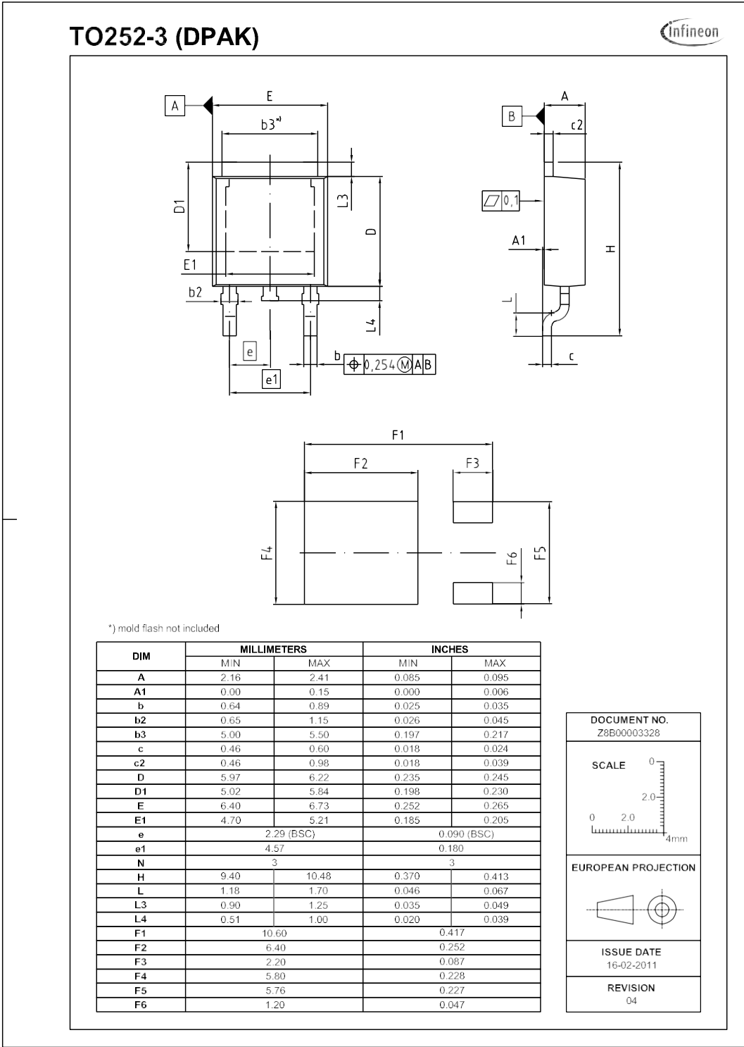
图 1 PG-TO252-3 外形图，尺寸单位为毫米
