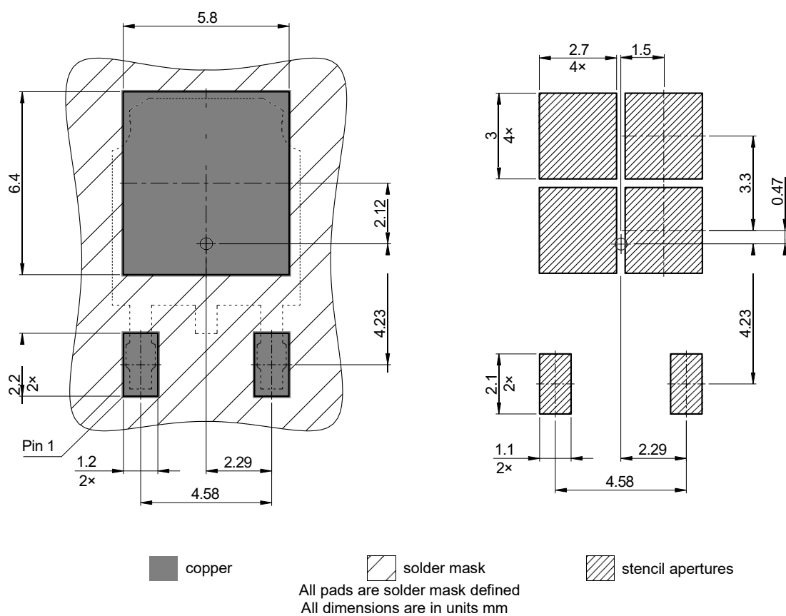
图 2 PG-TO 252 - 3封装图，尺寸单位为毫米
