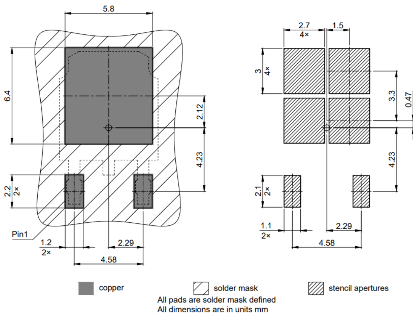
图 2 PG-TO 252 - 3封装图，尺寸单位为毫米
