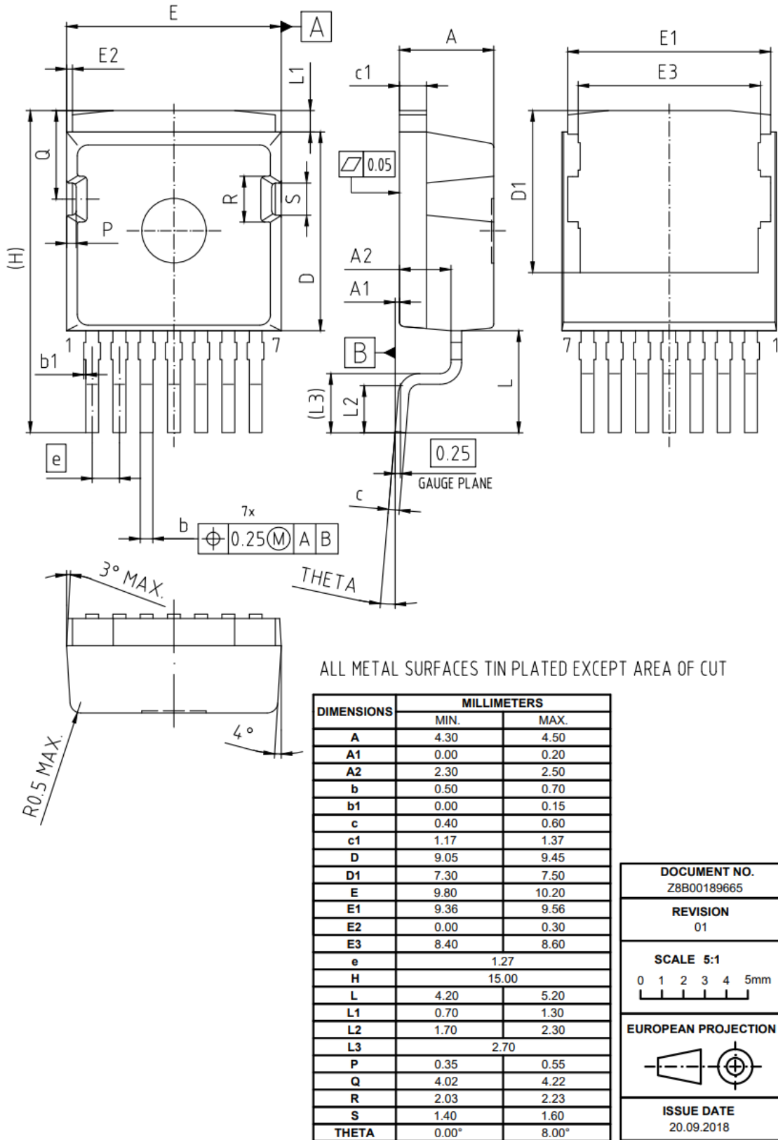
图 1 PG-TO263-7-11 外形图，尺寸单位为毫米
