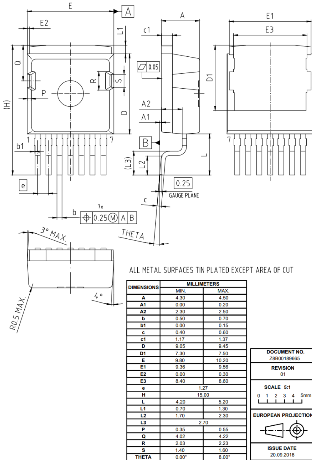
图 1 PG-T0263-7-11 外形图，尺寸单位为毫米
