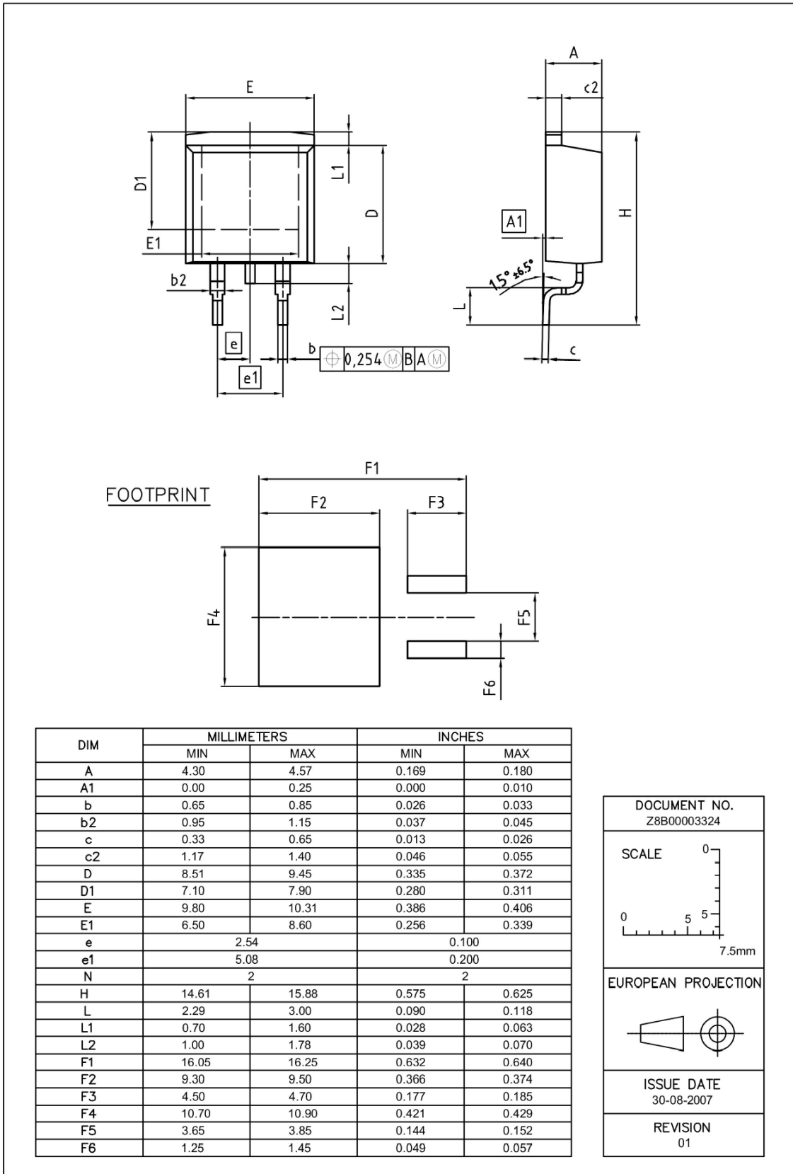
图 1 PG-T0263-3 外形图，尺寸单位为毫米/英寸
