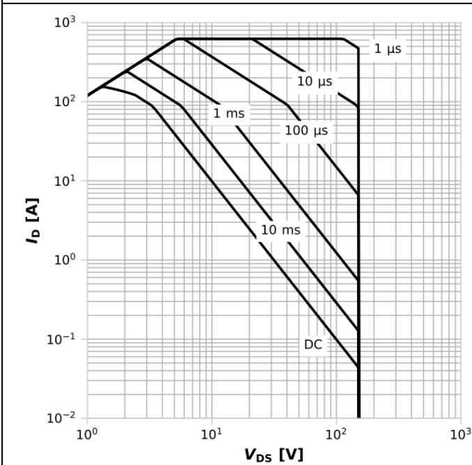
图3: 安全操作区
