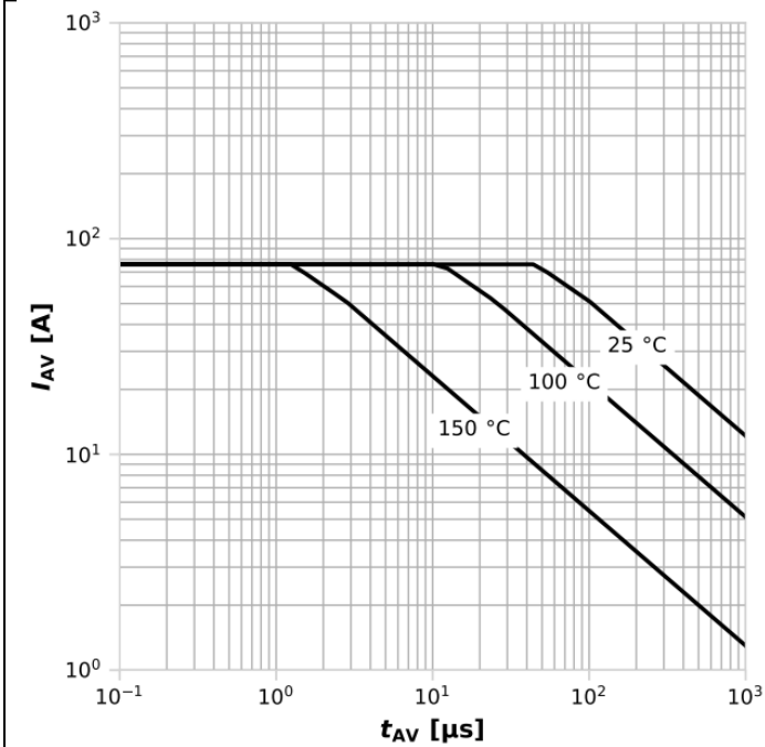
图 13: 雪崩特性
