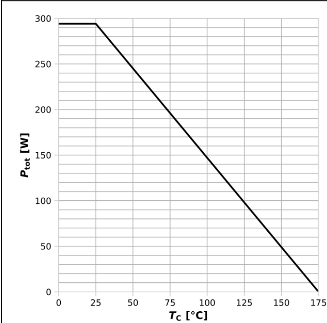
图1: 功率耗散
