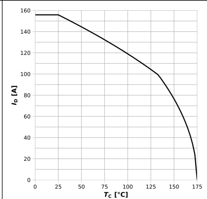
图2: 漏极电流
