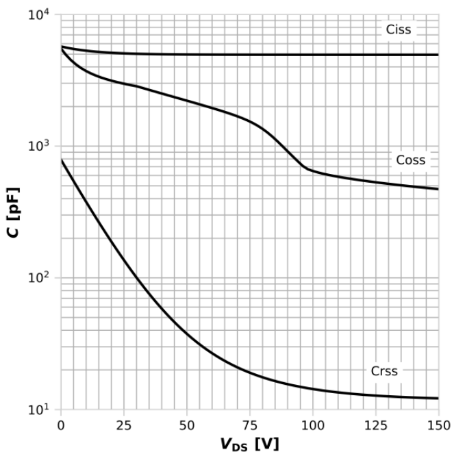
图11: 典型电容值
