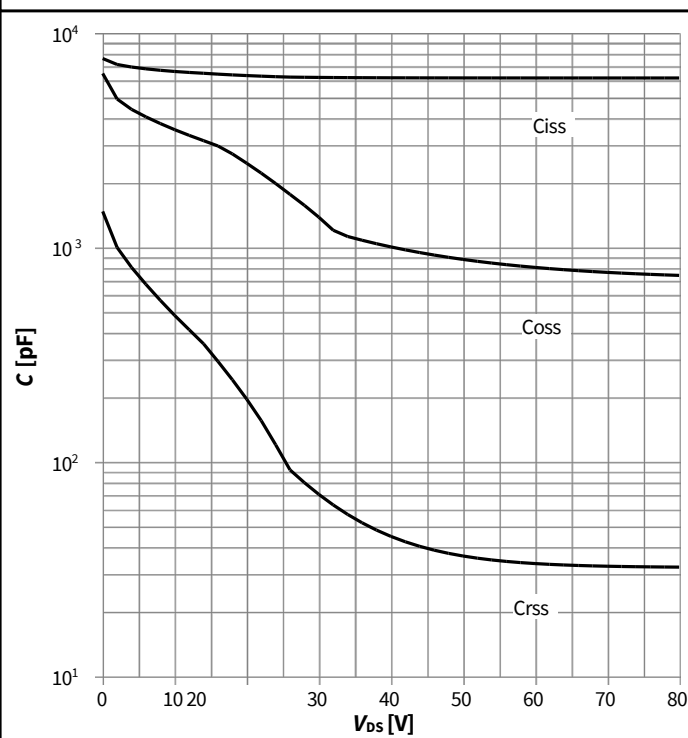
图 11: 典型电容值
