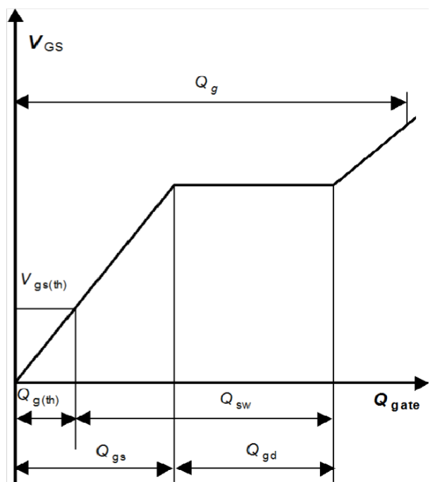
图 栅极充电波形
