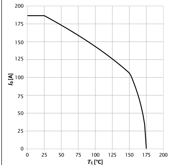
图 2: 漏极电流
