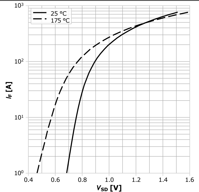
图 12：典型反向二极管的正向特性
