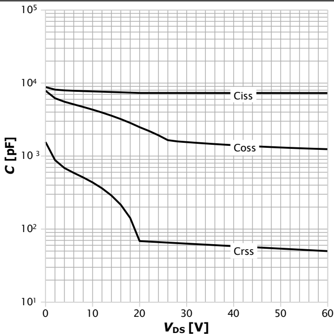
图 11：典型电容值
