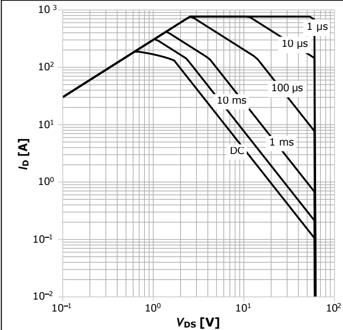
图 3: 安全操作区
