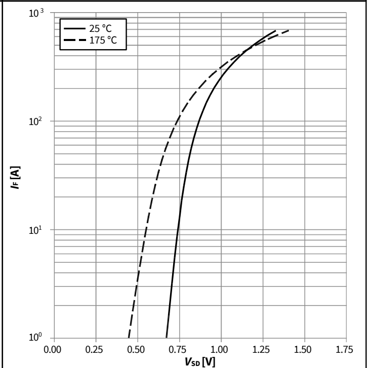
图 12：典型反向二极管的正向特性
