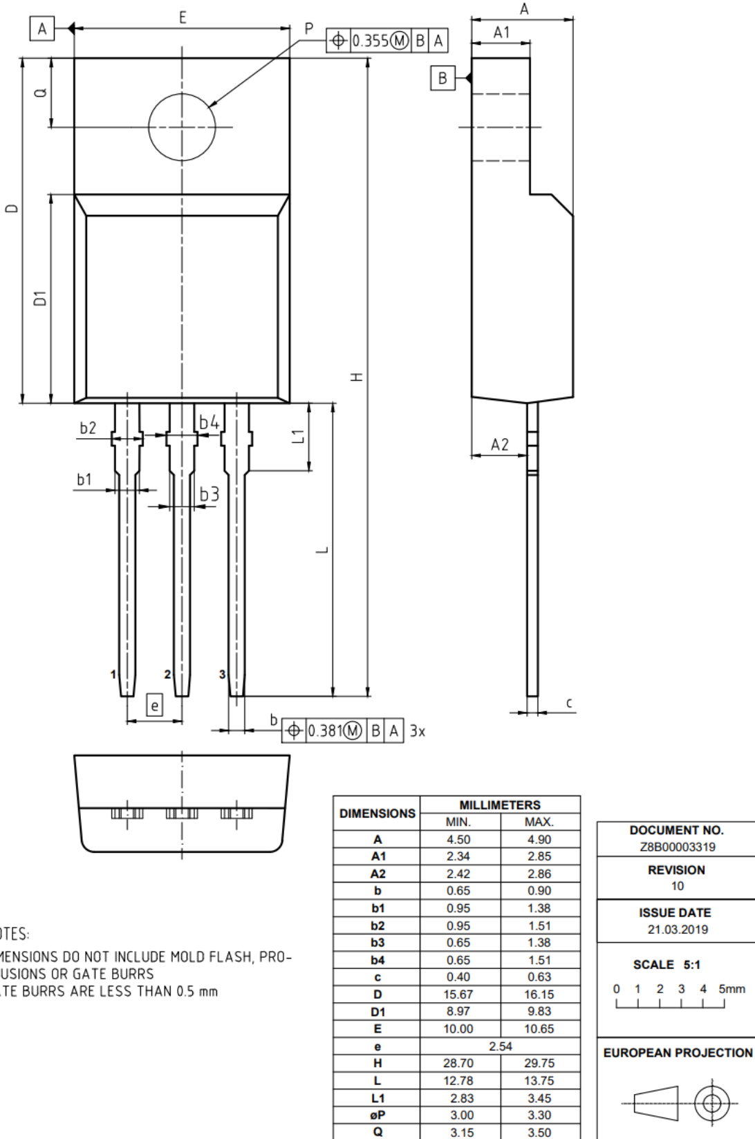
图 1 PG-T0220 FullPAK 封装外形图，尺寸单位为毫米
