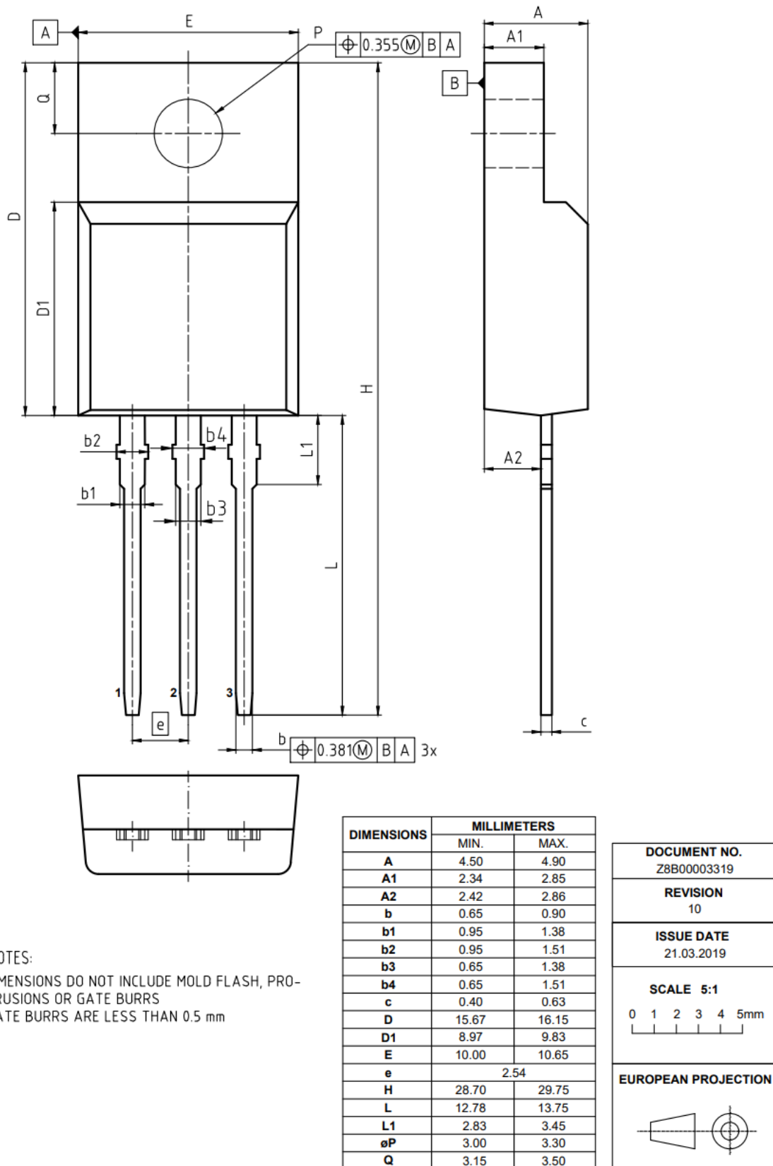
图 1 PG-TO220 FullPAK 封装外形图，尺寸单位为毫米
